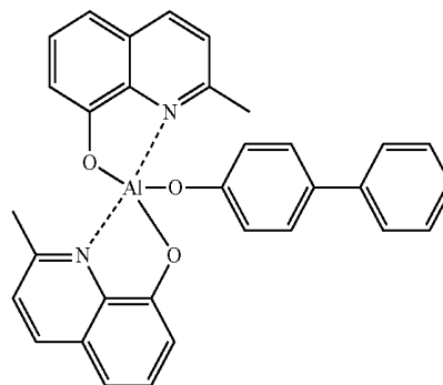
Balq
