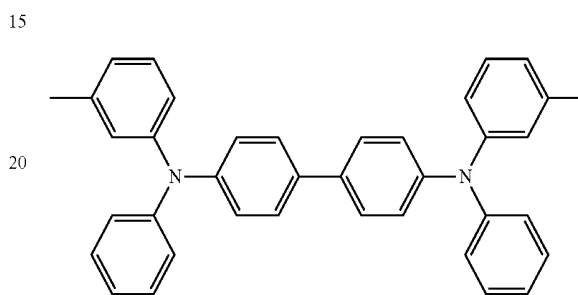
TPD
