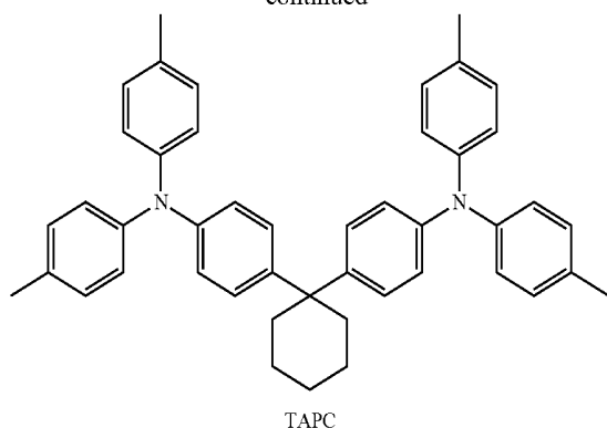
TAPC
